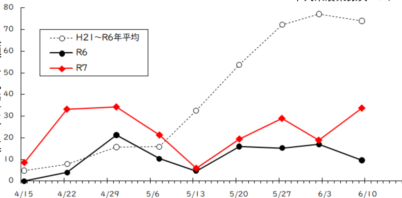
気温の推移(野市)
